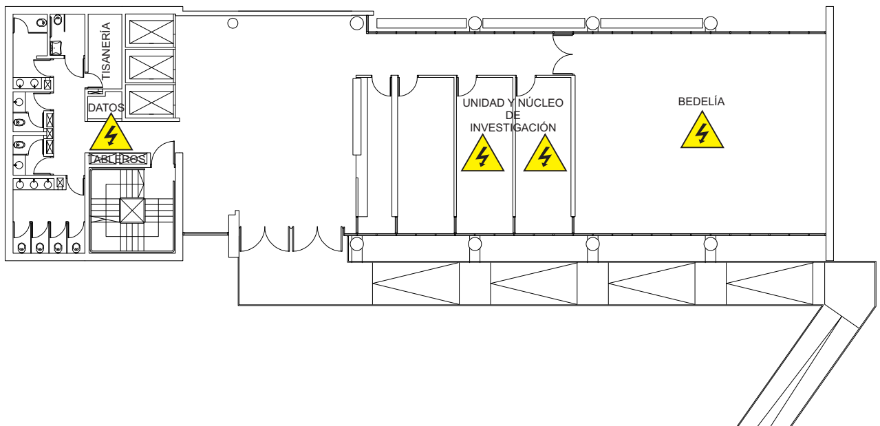
PLANTA BAJA
